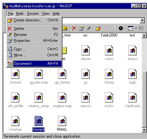
図 9: Winscp の終了
