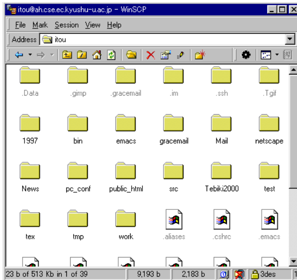
図 4: 接続画面
