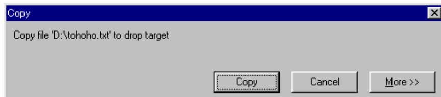
図 6: Copy の確認
