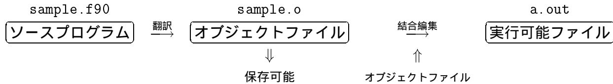
図 1: 実行可能ファイルの作成手順
