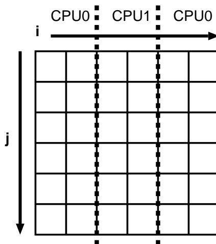
図 8: 配列の分割
