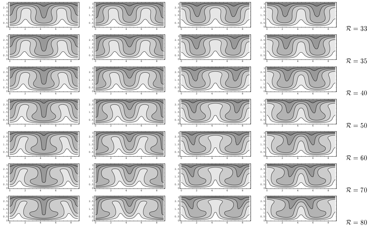
図 11: 他の非自明解 (等温場)
