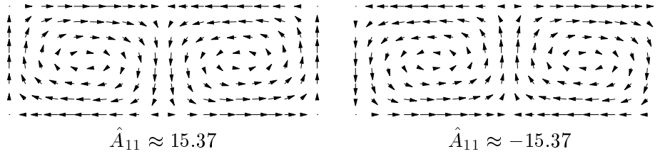
図 2: 自明解からの第 1 分岐解 (速度場)
