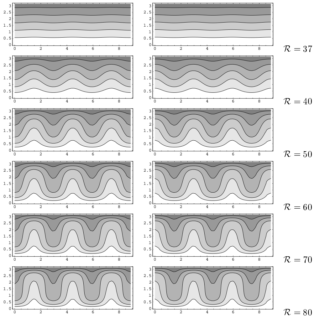
図 9: 自明解からの第 3 分岐解 (等温場)
