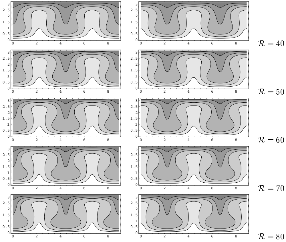
図 7: 自明解からの第 2 分岐解 (等温場) 続き
