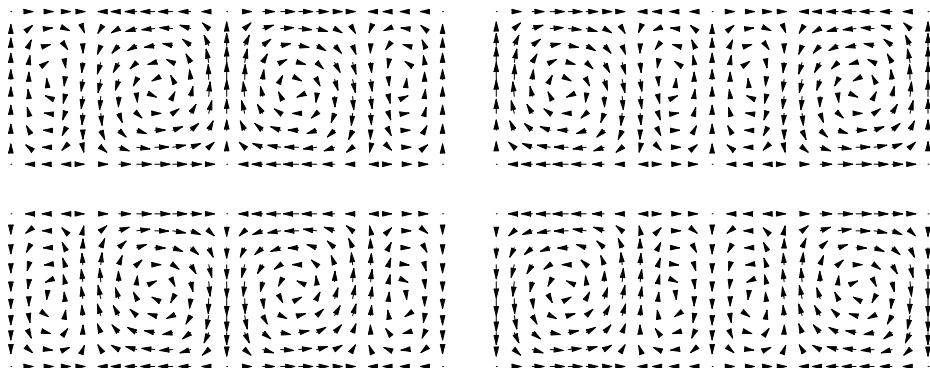
図 10: 他の非自明解 (速度場)
