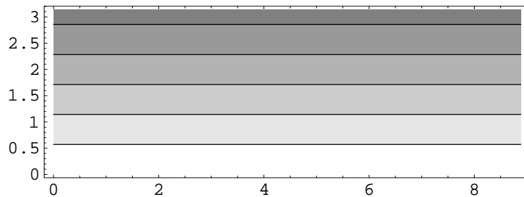
図 1: \Theta = 0 の時の等温場
