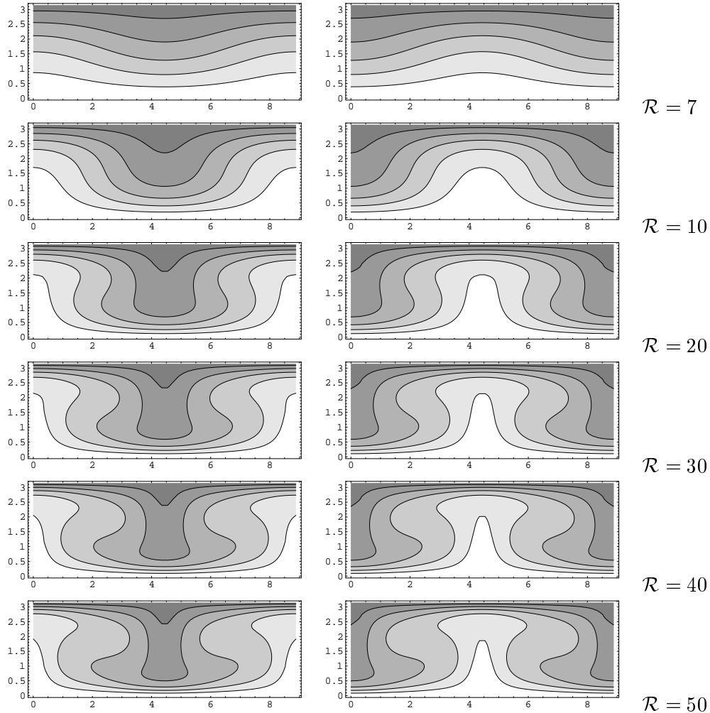
図 3: 自明解からの第 1 分岐解 (等温場)
