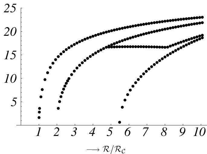
図 12: 検証に成功した非自明解
