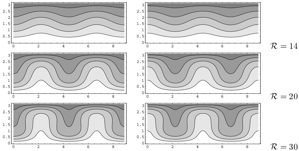
図 6: 自明解からの第 2 分岐解 (等温場)
