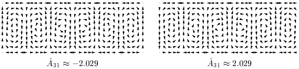
図 8: 自明解からの第 3 分岐解 (速度場)
