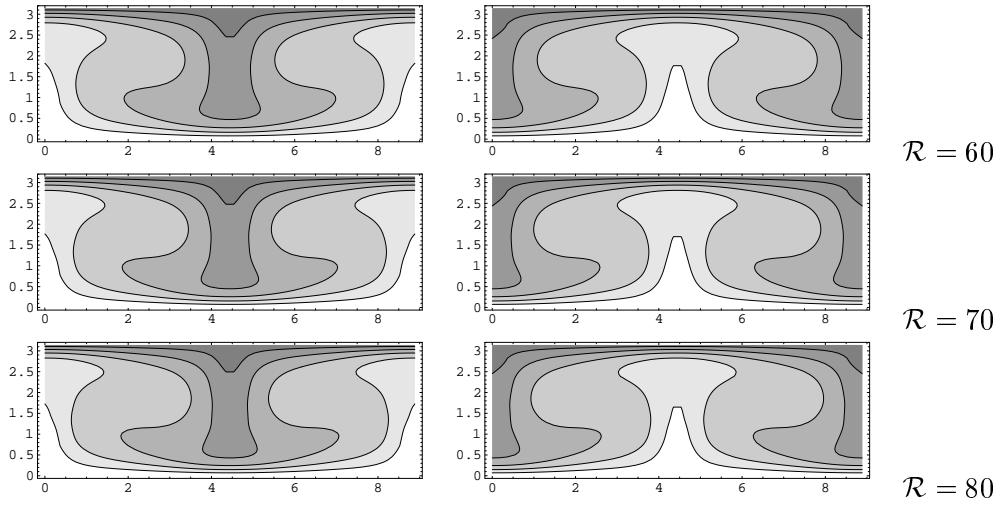
図 4: 自明解からの第 1 分岐解 (等温場) 続き
