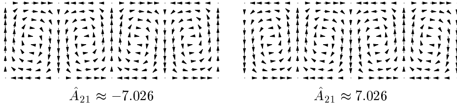
図 5: 自明解からの第 2 分岐解 (速度場)
