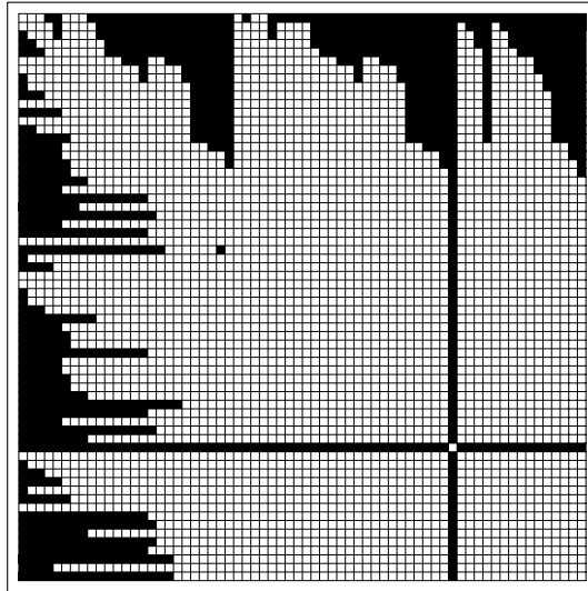
LU 分解後の行列の形
