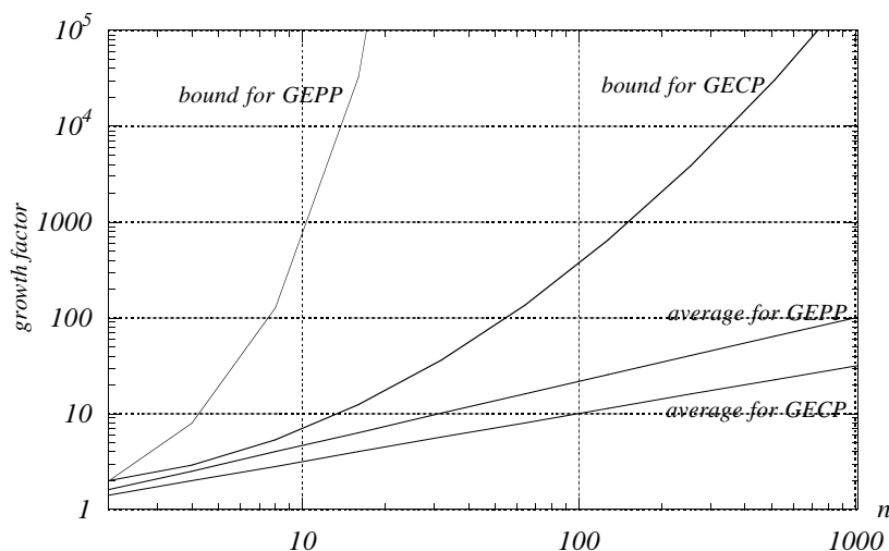
不安定因子の増大の様子
