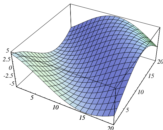
スケーリング前の行列
