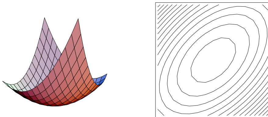
f(x) の形状と等高線図
